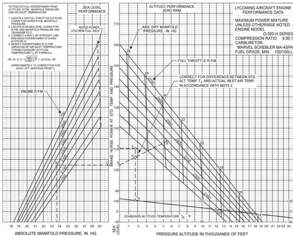
Slika 4. Dijagram performansi motora [4]
