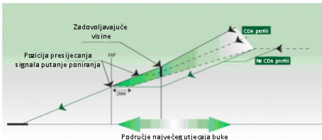
Slika 6 Profili prilaženja zrakoplova po konvencionalnoj i CDA metodi [9]
