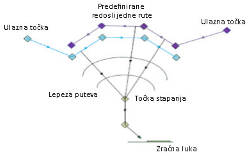
Slika 7 Struktura točke stapanja prometa [8]
