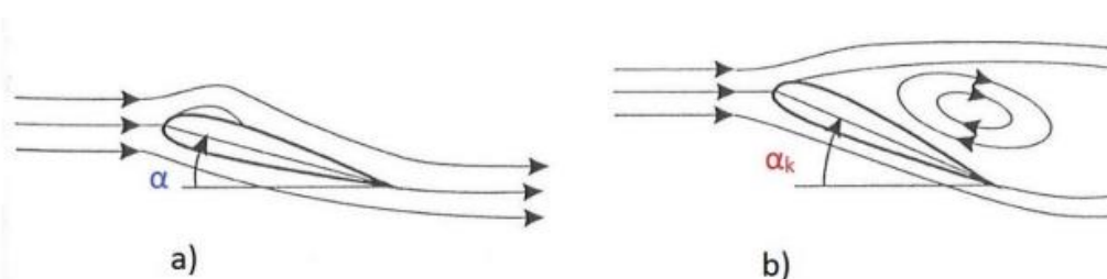
Slika 12. Mjehurasta zona odvajanja kod tankih aeroprofila s malim radijusom zakrivljenja nosa, a) umjeren napadni kut \alpha < \alpha_k , b) slom uzgona \alpha \geq \alpha_k
