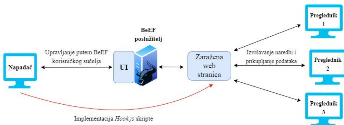
Slika 5. Način rada BeEF alata [27]
