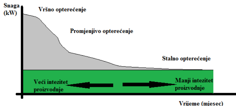
Dijagram 5. Krivulja trajanja opterećenja
