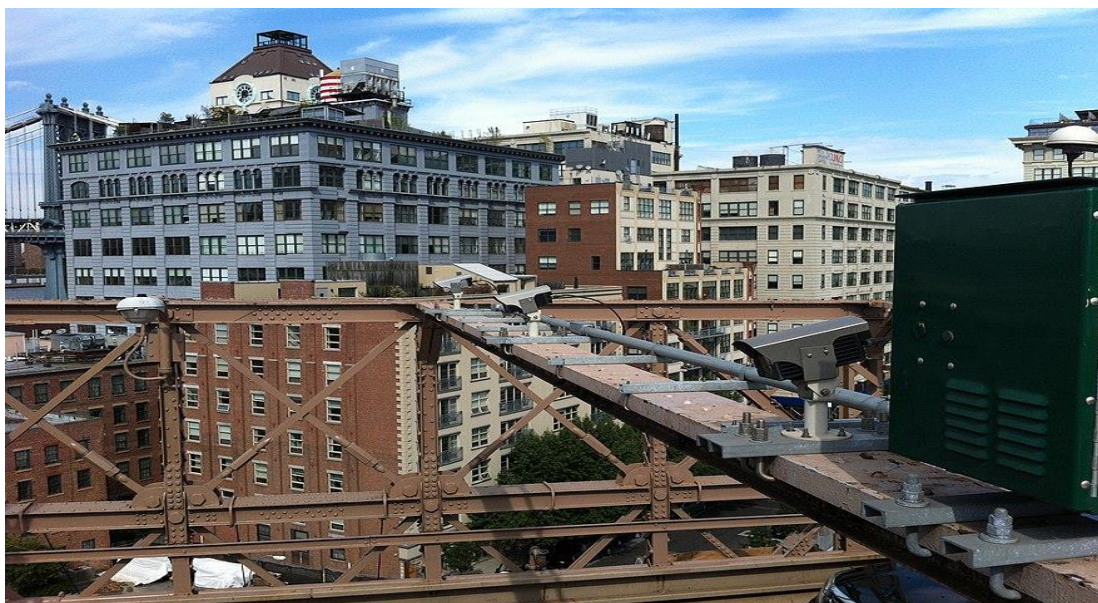
Slika 4. ANPR sustav kamera na Brooklyn Bridgeu u New Yorku
