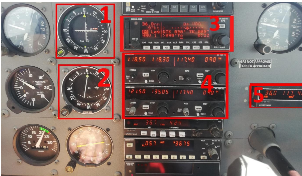
Slika 15. Dio instrument ploče zrakoplova 9A-DAD
