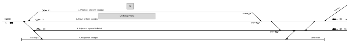
Slika 6. Shema kolodvora Velika Gorica
