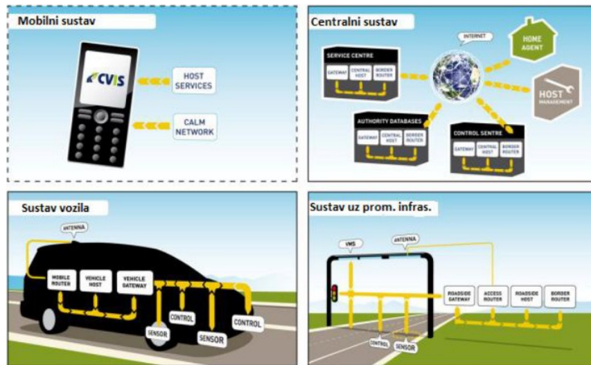
Slika 9. CVIS arhitektura
