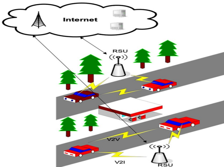
Slika 8. DSRC arhitektura
