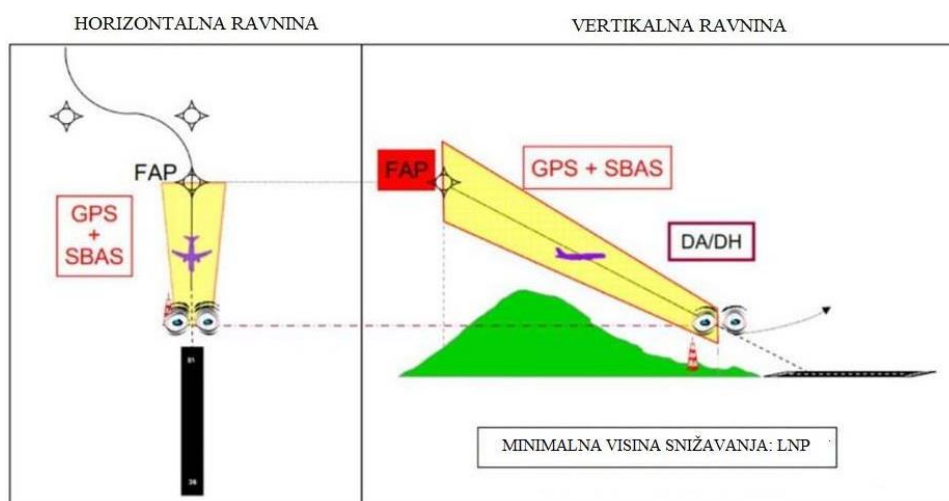
Slika 4.8. Prikaz generalnog APV - SBAS postupka prilaznja, [8]
