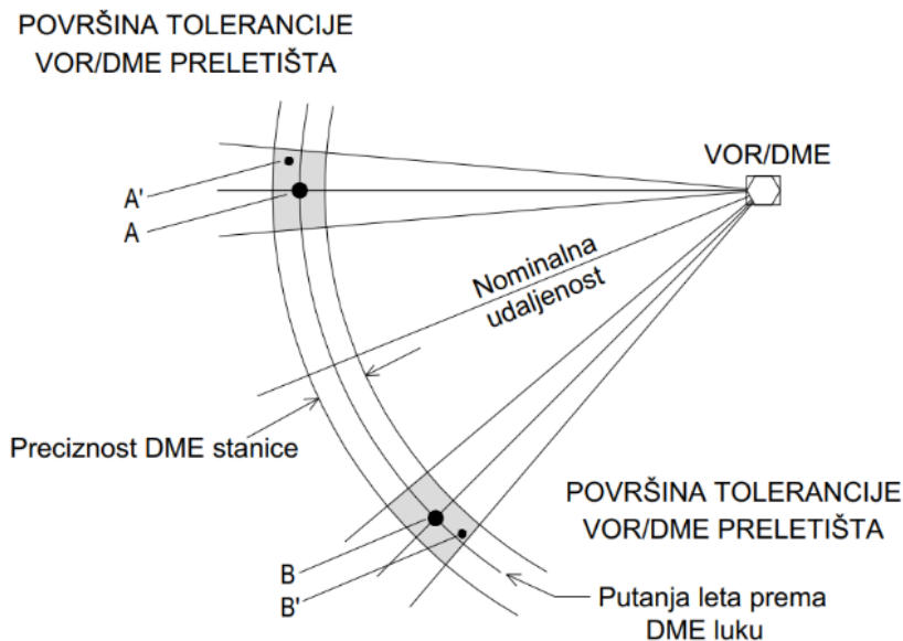
Slika 5.1. Prikaz preletišta formirano VOR/DME stanicom
