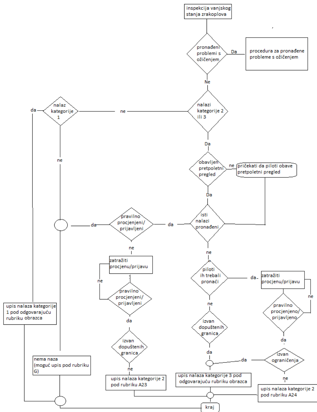
Slika 4 Dijagram toka prepoletnog pregleda zrakoplova, izvor: [8]
