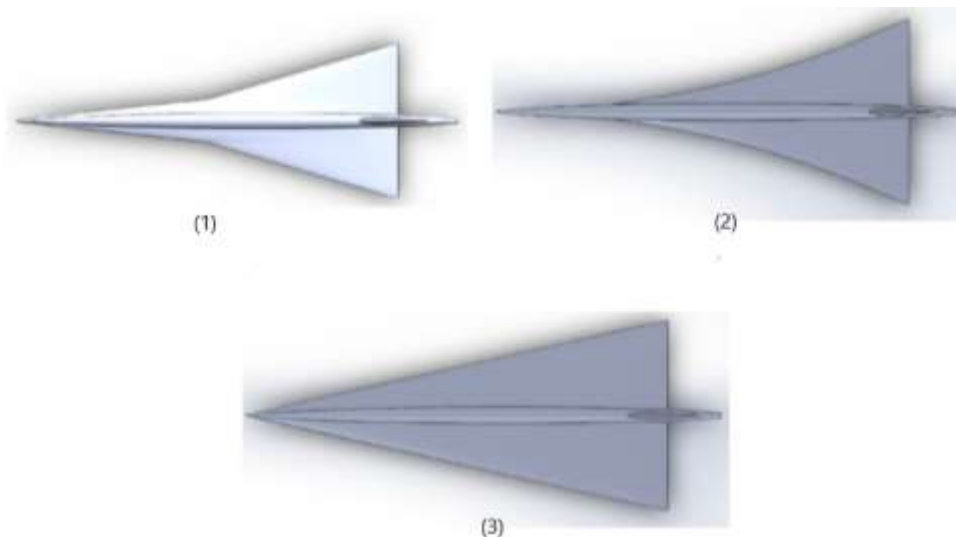
Slika 29. Zrakoplov s: 1) delta krila sa strake površinom, 2) delta krila s povijenim napadnim bridom, 3) ravna delta krila [21]
