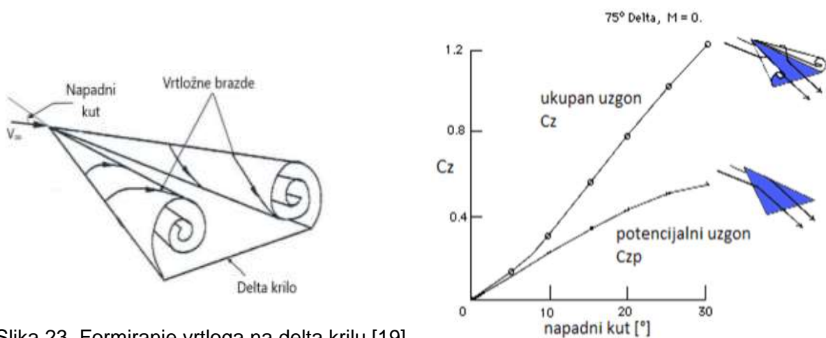
Slika 23. Formiranje vrtloga na delta krilu [19]
