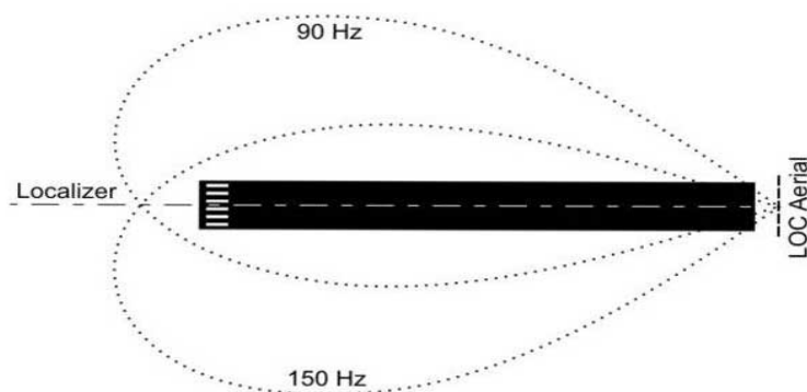
Slika 6. Signali koje prenosi Localizer . [4]
