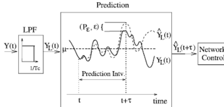
Slika 5. Okvir predviđanja mrežnog prometa, [15]
