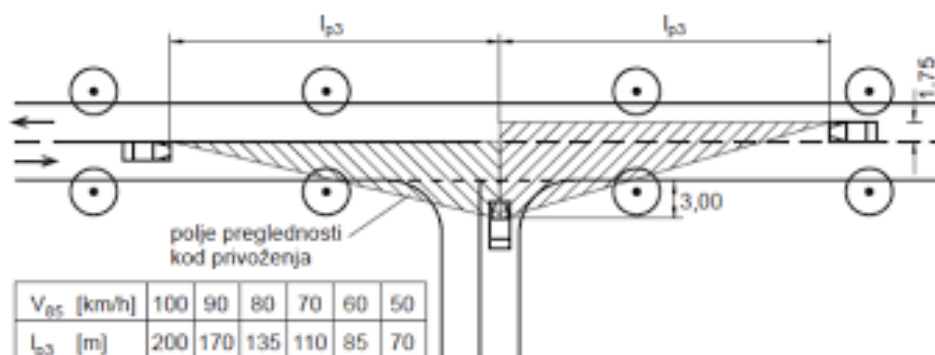
Slika 3. Privozna preglednost [2]
