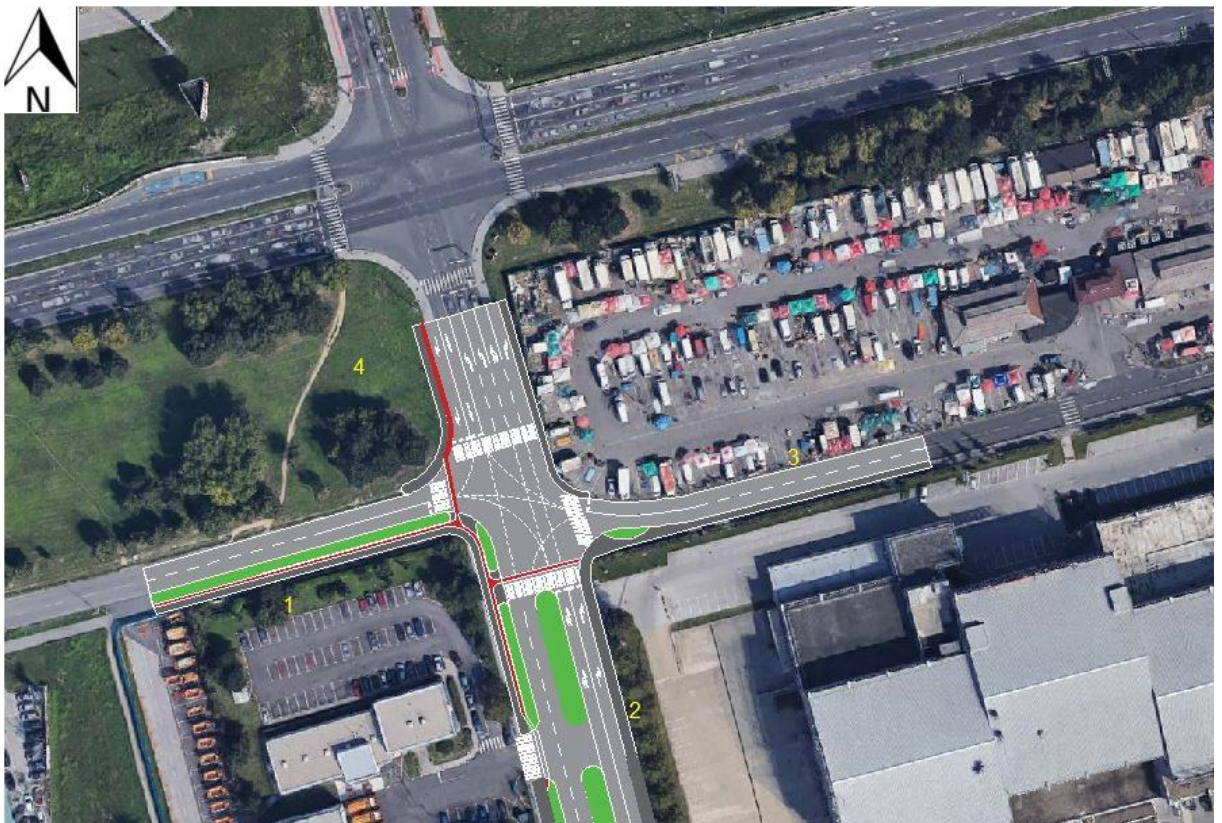
Slika 18. Prvo varijantno rješenje raskrižja
