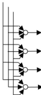
Slika 10: Primjer jednodimenzionalne ljestvičaste mreže, [11]
