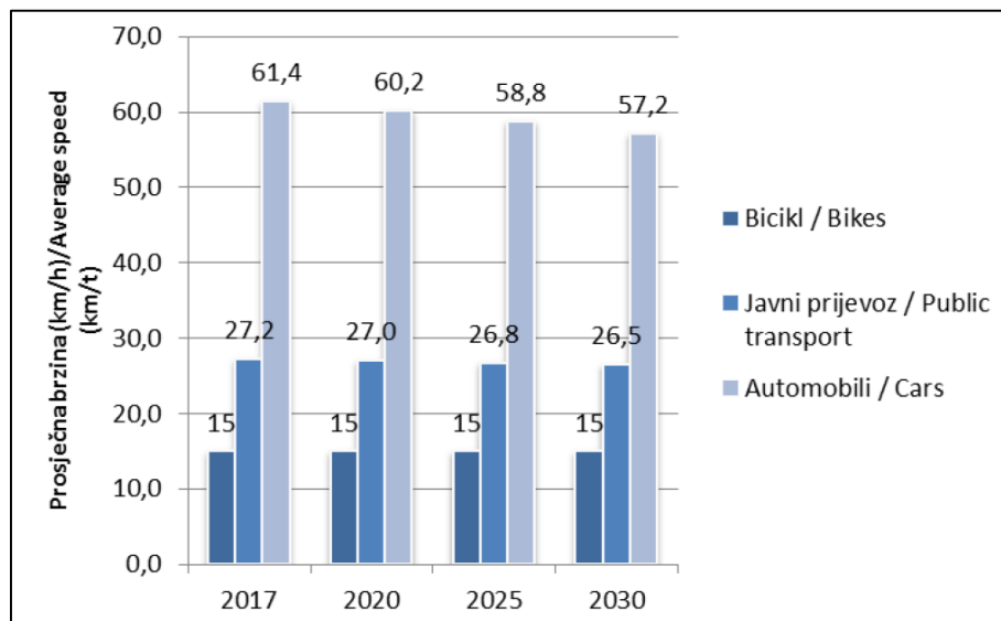
Slika 2.6. Prosječna brzina (km/h) na radni dan unutar područja Masterplana, 2017., 2020., 2025. i 2030., [5]
