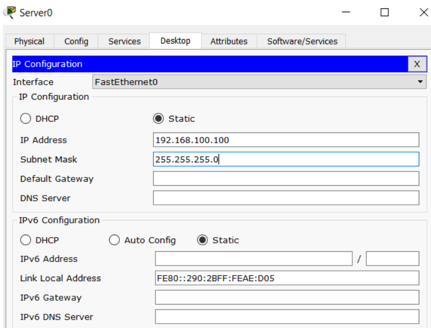
Slika 8 : Adresiranje servera
