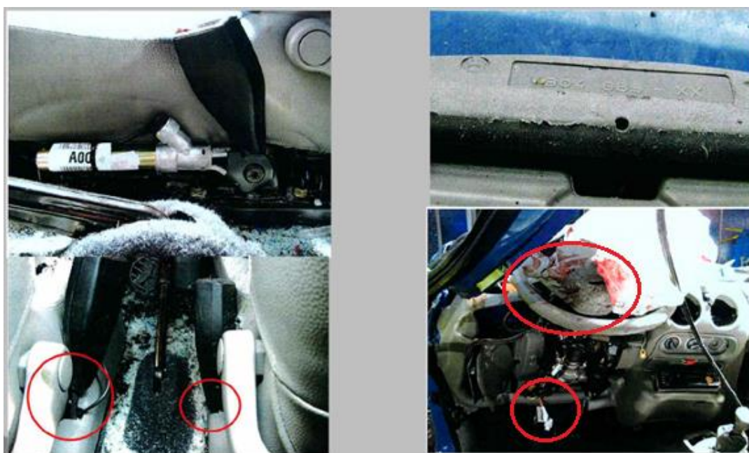
Slika 9. Označavanje tragova na unutrašnjosti vozila
