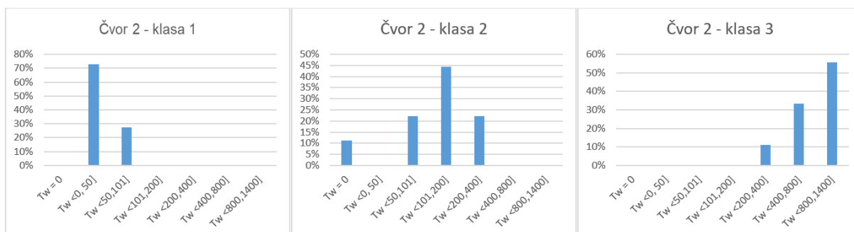
Slika 28. Postotak paketa koji moraju čekati u 2. čvoru
