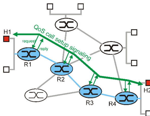
Slika 22. IntServ mehanizam, [40]
