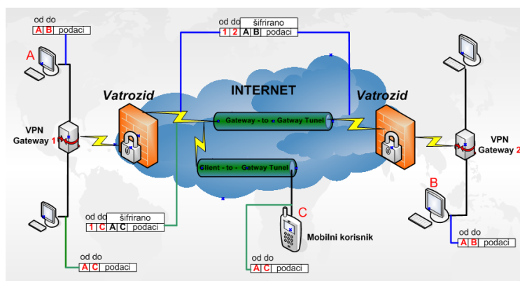
Slika 21. Tuneliranje kroz VPN mrežu
