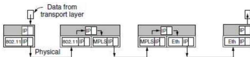
Slika 20. Proces obrade paketa [38]
