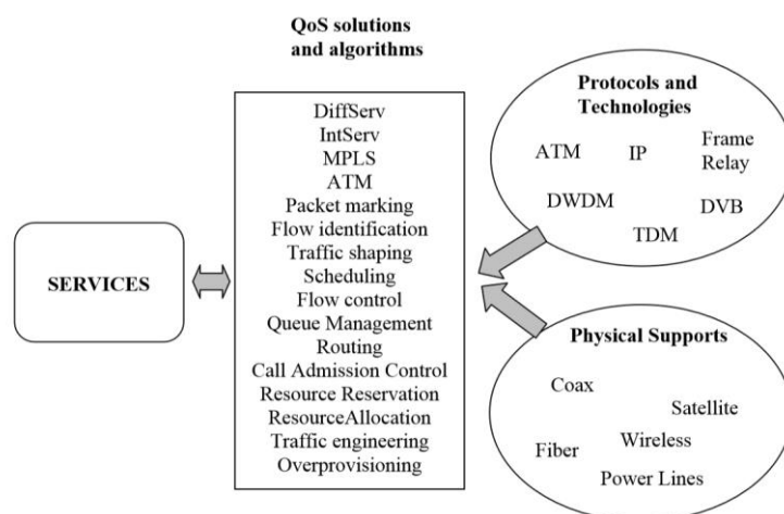
Slika 15. Heterogenost mreže, [37]
