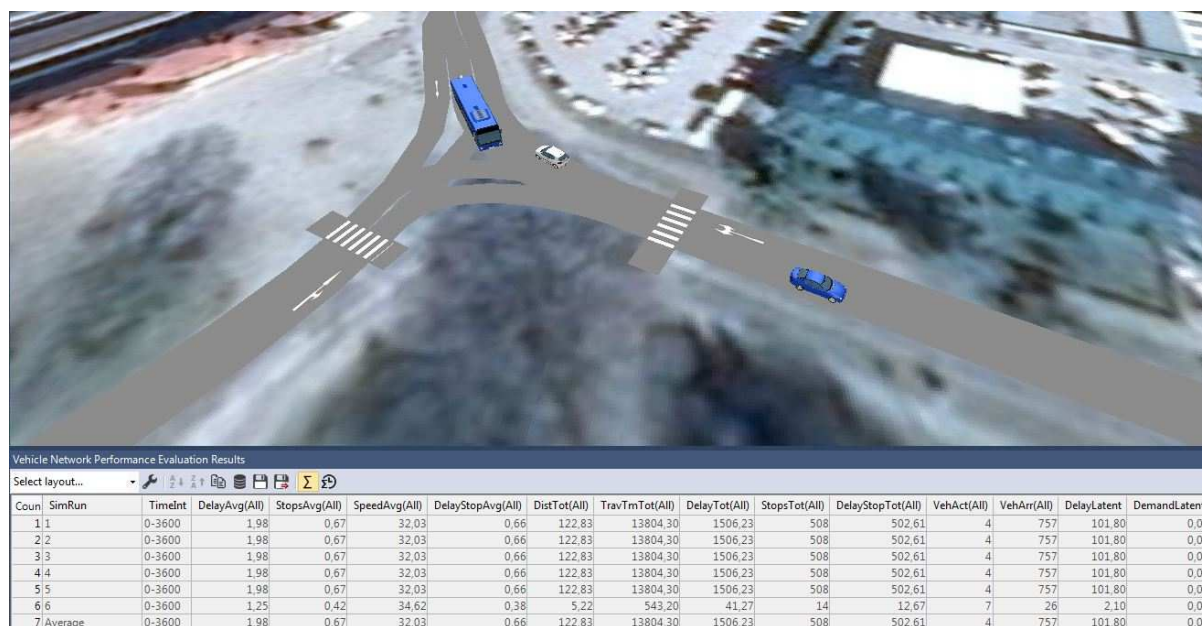
Slika 56. Simulacija postojećeg stanja raskrižja Kolodvorske ulice i Ulice Ivana Meštrovića
