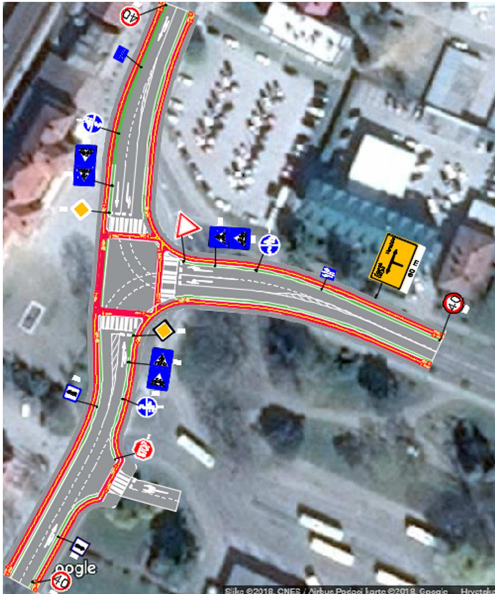
Slika 45. Prikaz rekonstruiranog raskrižja Kolodvorske ulice i Ulice Ivana Meštrovića
