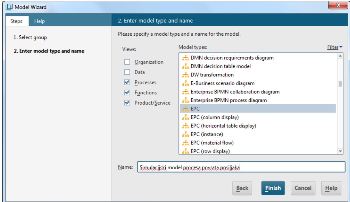
Slika 7: Kreiranje modela
