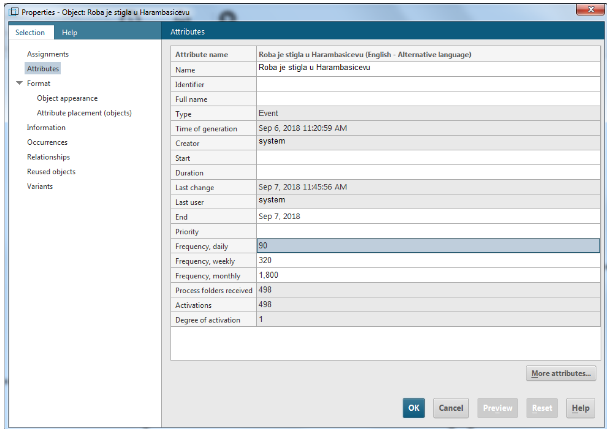
Slika 8: Kreiranje događaja
