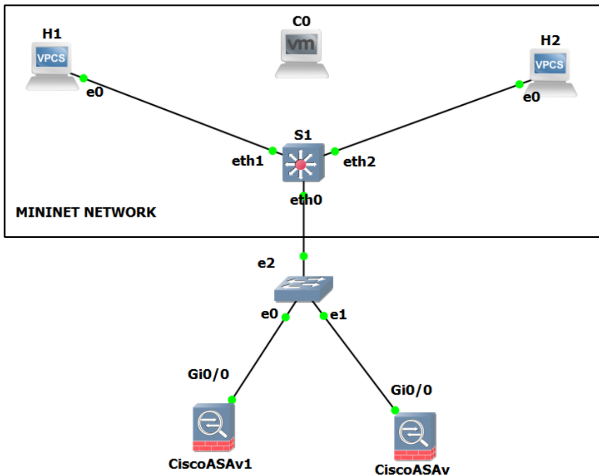
Slika 14. Logički prikaz simuliranog sustava
