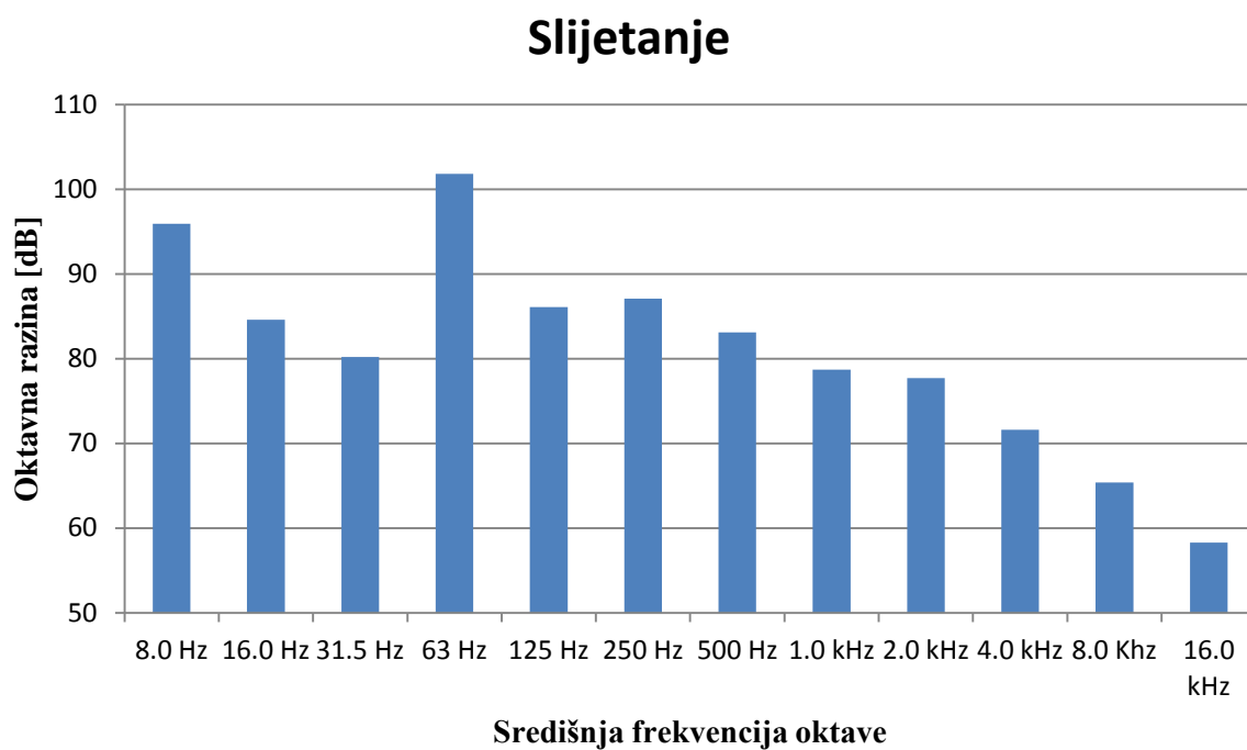
Slika 24. Grafikon unutarnjeg oktavnog mjernja buke zrakoplova CL-415 na slijetanju
