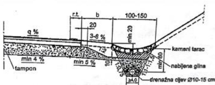
Slika 23 Vrsta rigola - segmentni
