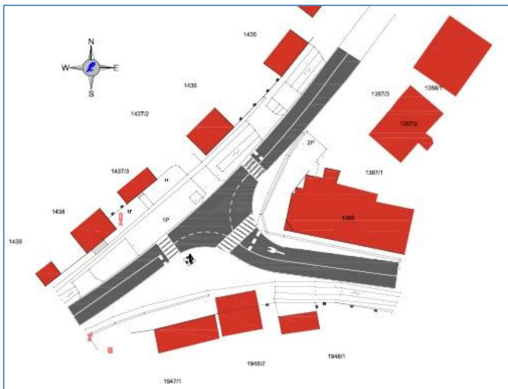
Slika 23: T-raskrižje idejni
