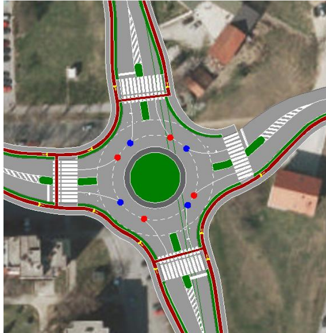
Slika 33. Konfliktni točke na raskrižju s kružim tokom prometa
