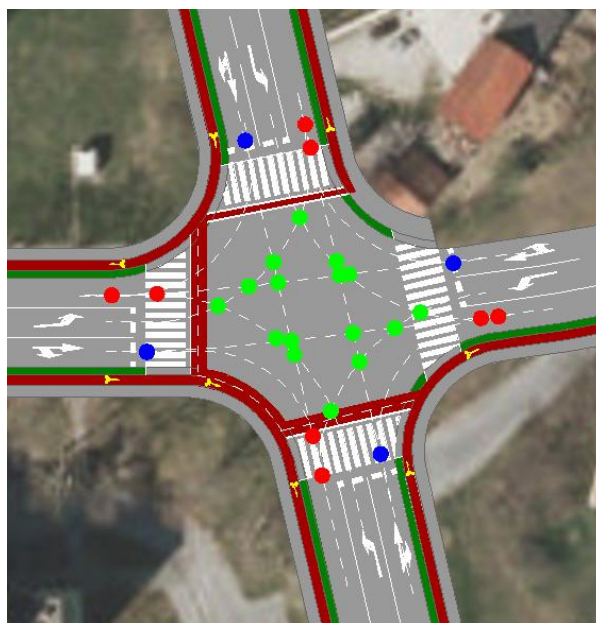
Slika 34. Konfliktni točke na četverokrakom raskrižju i raskrižju upravljanoj prometnim svjetlima
