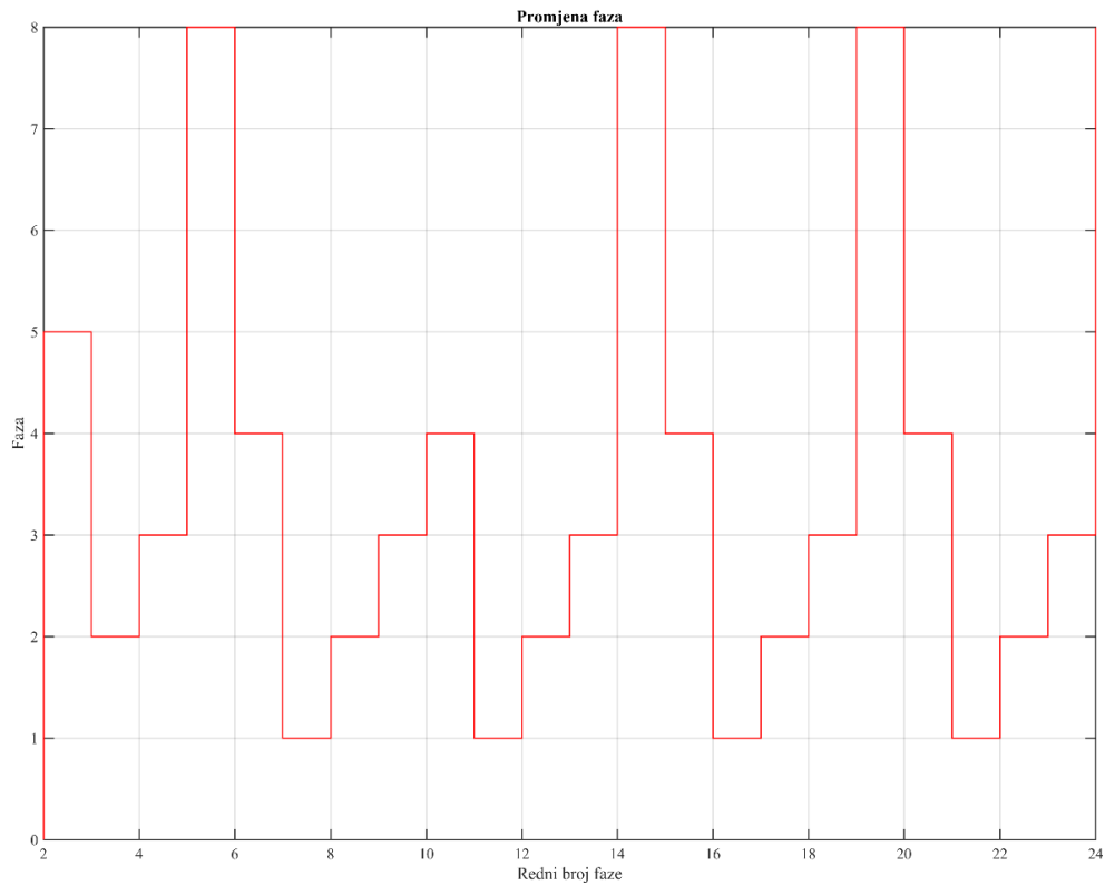
Slika 20. Prikaz izmjene faza korištenjem strukture NEMA i implementiranog neizravnog sustava upravljanja
