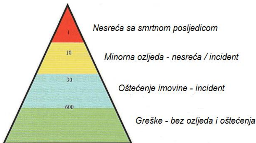
Slika 10. Heinrichova piramida [4]
