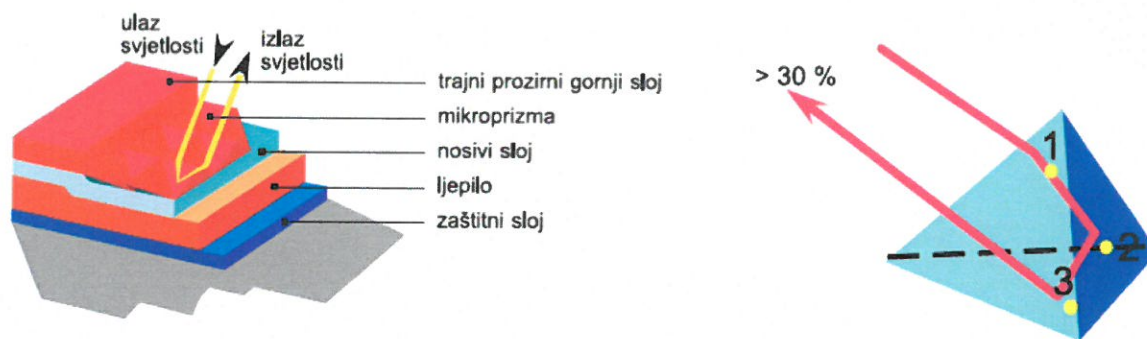
Slika 7. Struktura folije i način reflektiranja klase III, [12]
