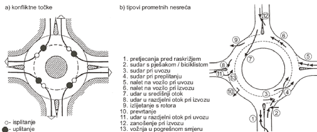
Slika 2.9. Konfliktne točke i tipovi prometnih nesreća raskrižja s kružnim tokom prometa, [1]
