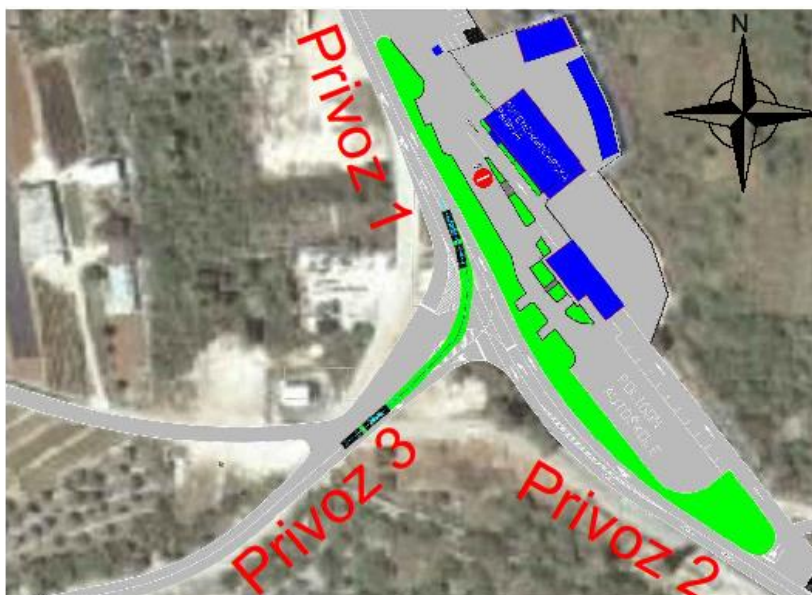
Slika 4.6. Provjera trajektorije mjerodavnog vozila na Ž6222
