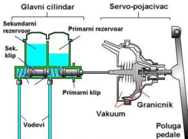
Slika 13. Servo uređaj[21]
