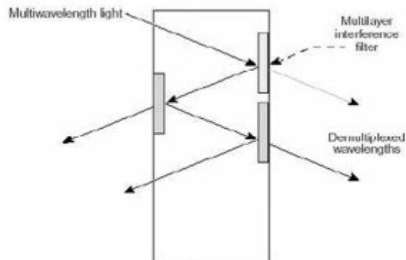
Slika 19. Interferencijski filter
