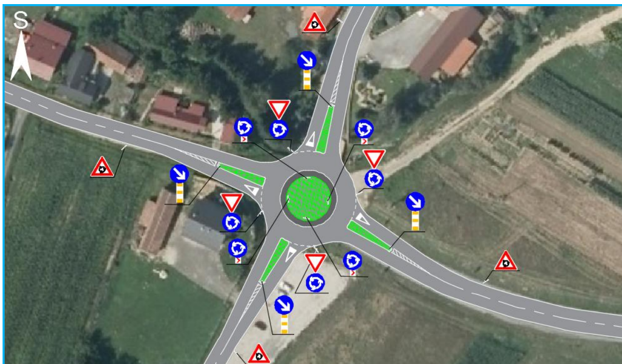
Slika 27. Idejno rješenje raskrižja 1 Izvor kartografske podloge: [7]
