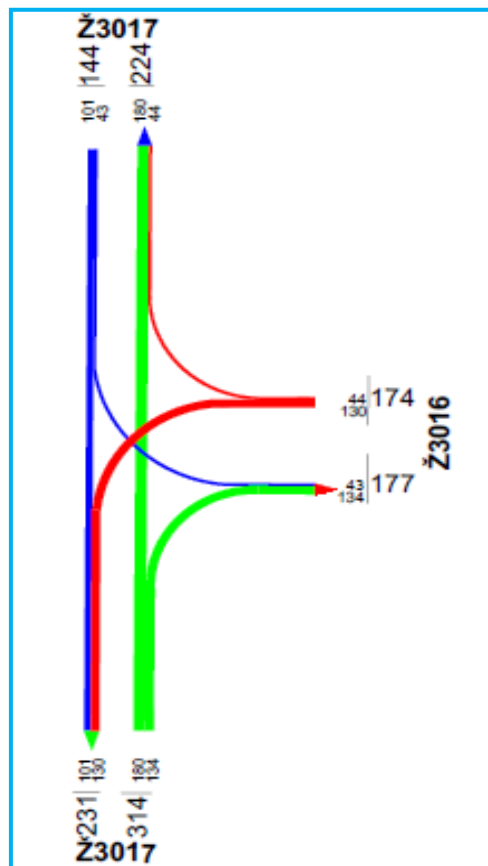
Slika 24. Distribucija satnog prometa na raskrižju 2 u popodnevnom vršnom satu
