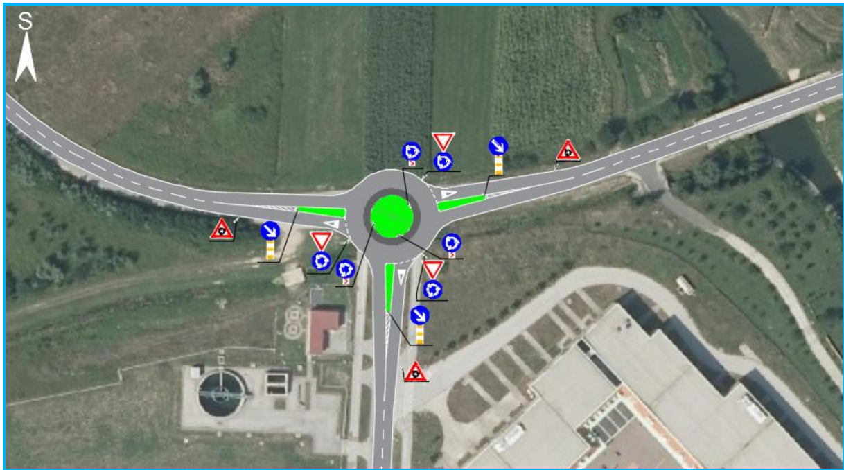
Slika 31. Idejno rješenje raskrižja 3
