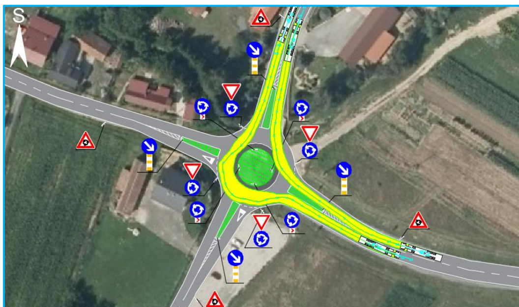
Slika 28. Trajektorija provoženja mjerodavnog vozila na raskrižju 1
