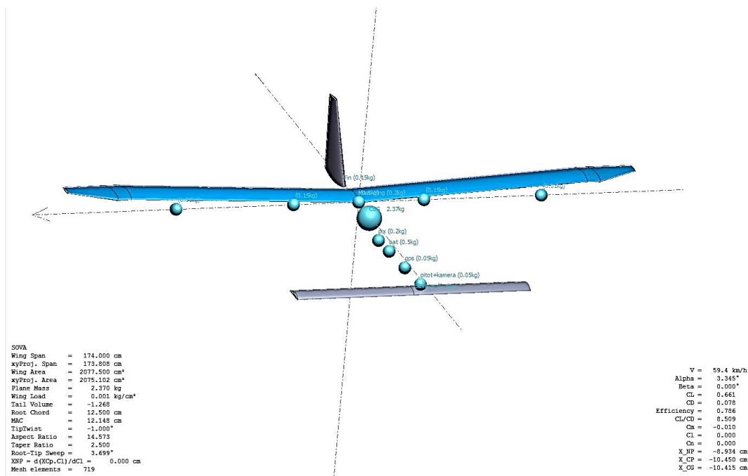
Slika 6. Aproximacija trupa letjelice točkastim masama u XFLR5 4
