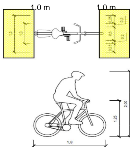
Slika 4. Prometni profil
