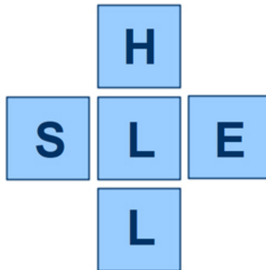
Slika 4. Shematski prikaz SHELL modela [18]
