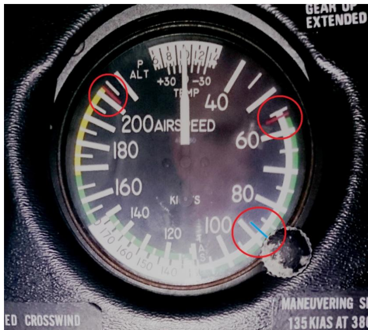
Slika 4: Brzinomjer zrakoplova PA-44, [4]
