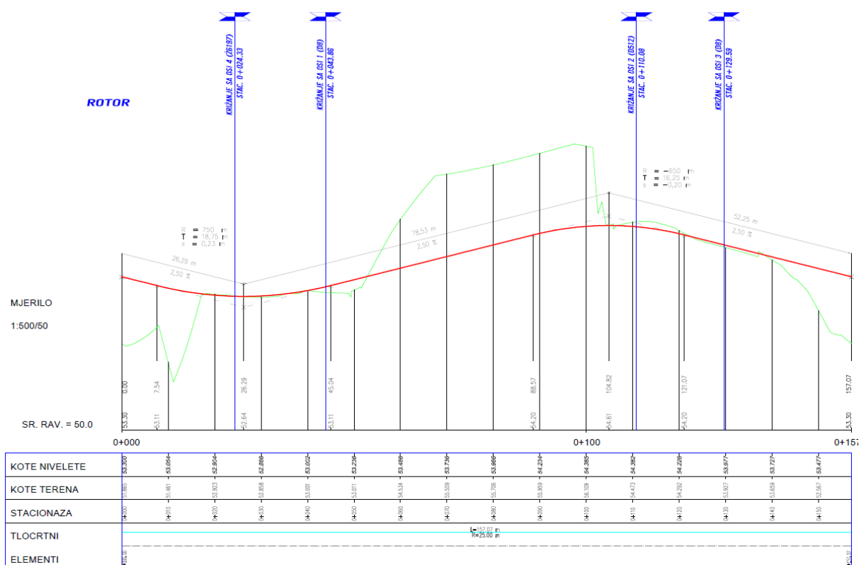
Slika 25. Uzdužni profil rotora, [10]
