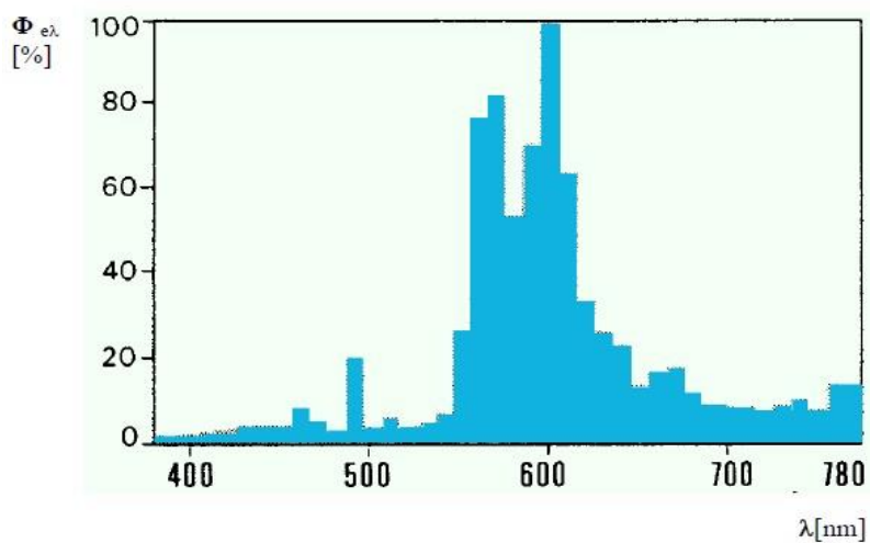
Slika 3. - Linijski spektar
