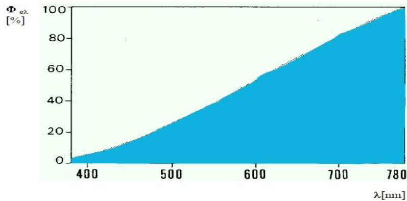
Slika 2. - Kontinuirani spektar
