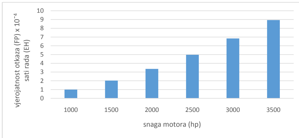
Dijagram 1. Vjerovatnost otkaza klipnog motora u odnosu na snagu (RPM=konst.)
