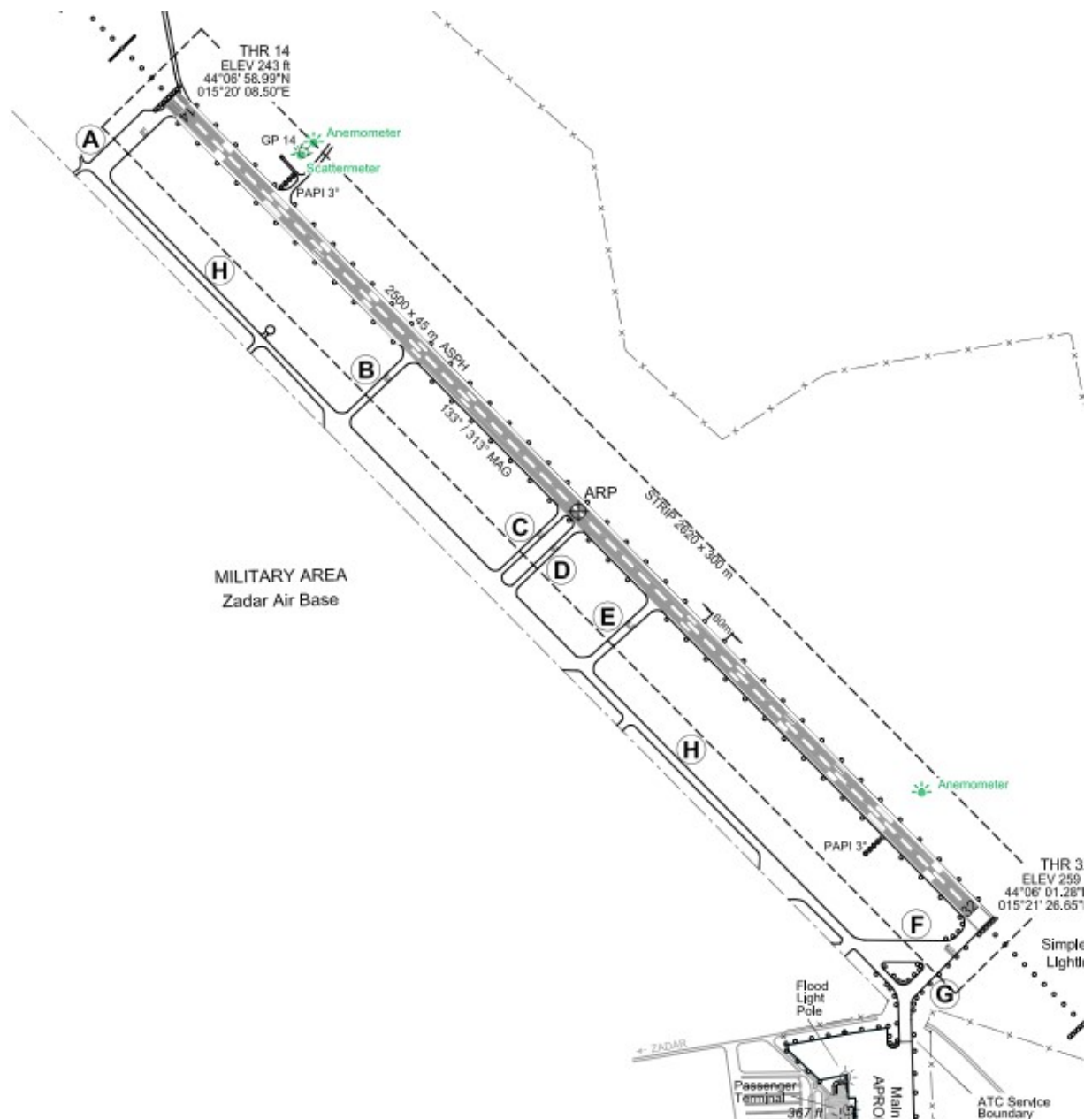
Slika 48. Shematski prikaz označavanja manevarske površine zračne luke Zadar na i oko staze 14-32
