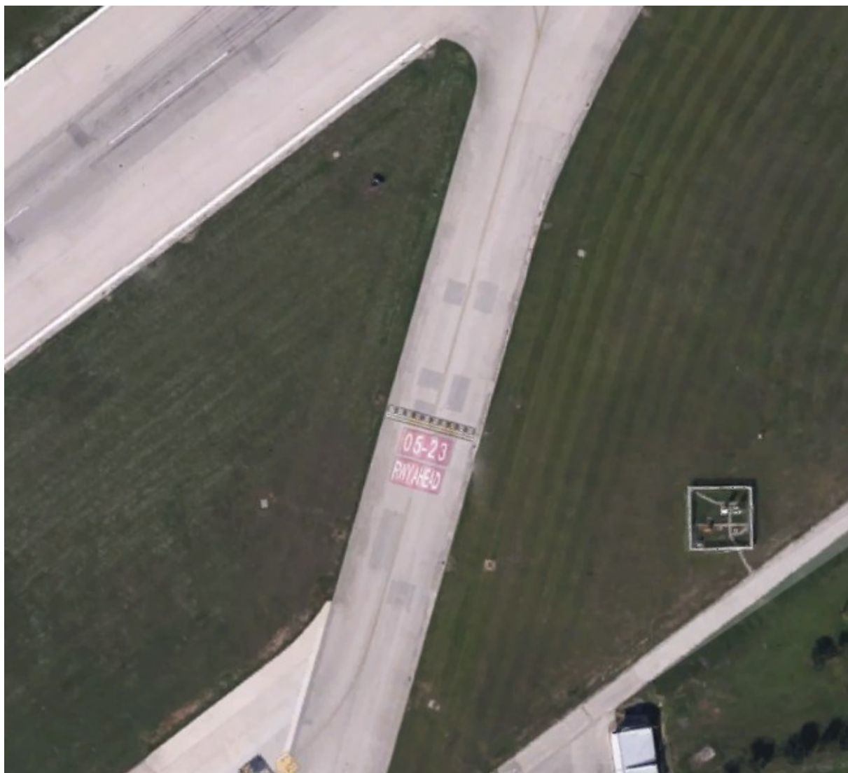
Slika 38. Oznake staze za vožnju zračne luke Split
