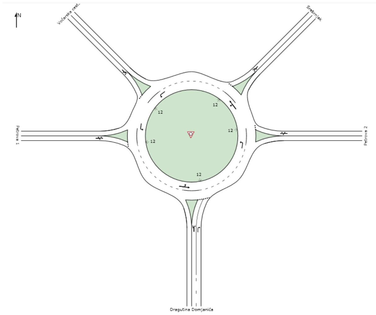
Slika 22. Geometrijski prikaz kružnog raskrižja Ul. Dragutina Domjanića – Petrova ulica – Srebrnjak – Voćarska ulica unutar SIDRA INTERSECTION programskog paketa.
