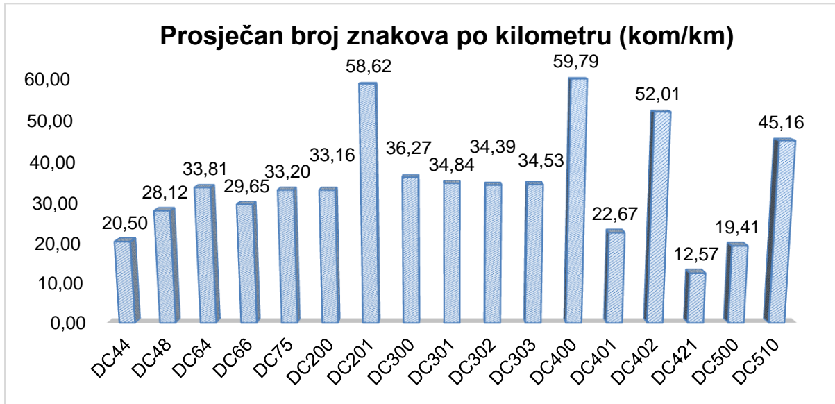
Grafikon 1. Prosječan broj znakova po kilometru na dionicama državnih cesta u Istarskoj županiji
