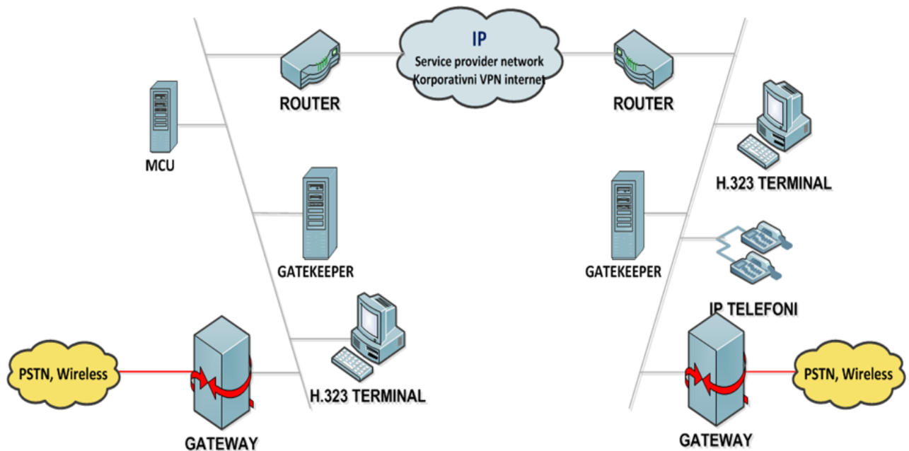
Slika 9. H.323 arhitektura. Preuzeto od [11].
