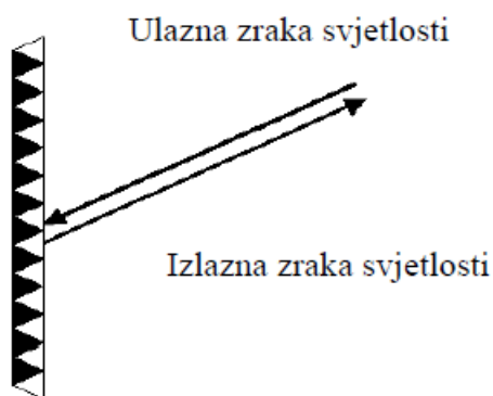
Slika 21. Retrorefleksija
