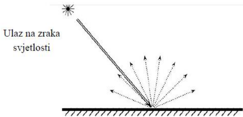
Slika 20. Difuzna refleksija
