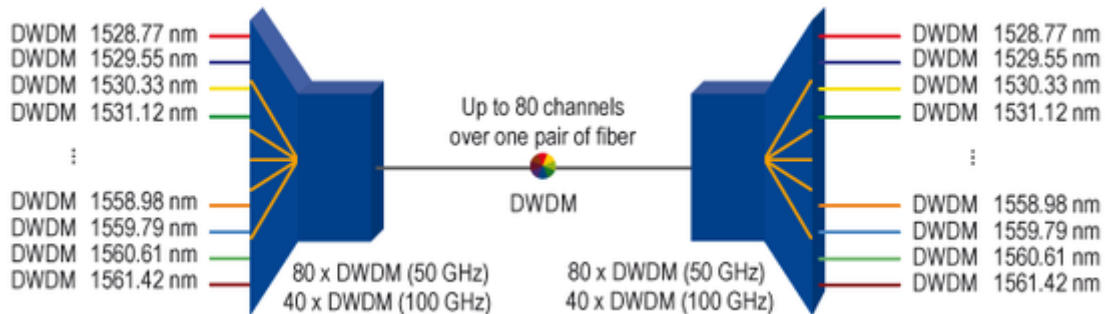
Slika 3. 80 kanalni dvosmjerni DWDM sustav
