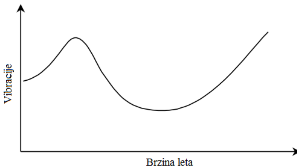
Slika 36. Dijagram utjecaja brzine leta na pojavu vibracija u kabini helikoptera.
