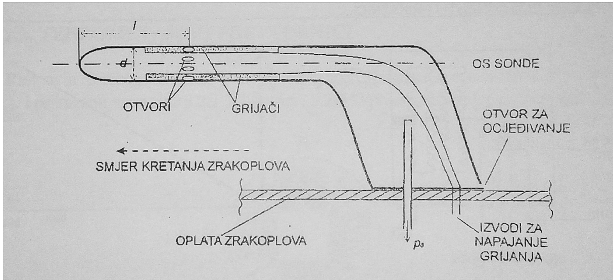
Slika 5. Statička sonda
