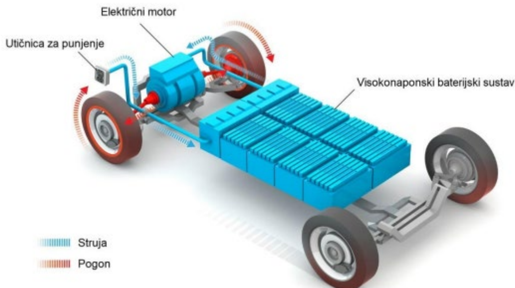
Slika 9. Princip rada električnog vozila
